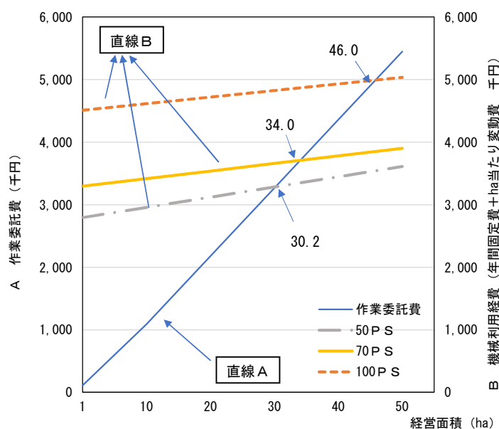
図－１ トラクターの作業委託費と機械利用経費 （自動操舵装置有り）の比較
