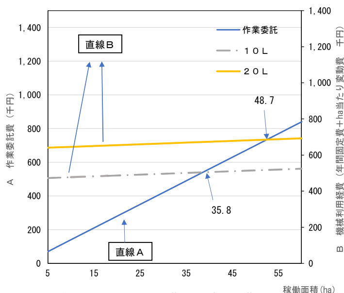
図－4 ドローンの作業委託費と機械利用費用との比較
