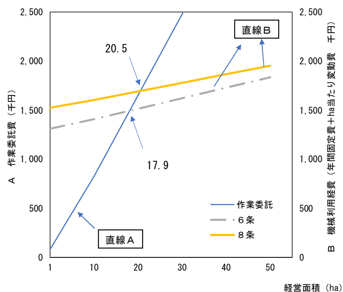
図－2 田植機の作業委託費と機械利用経費（直進アシスト機能付き）の比較
