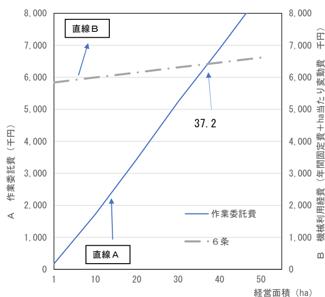
図－3 コンバインの作業委託費と機械利用費（自動運転アシスト機能付き・有人）の比較
